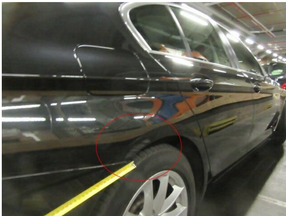
Bild 10 : Seitenteil hinten rechts, eingedellt, instandsetzen und lackieren mit Lackaufbau
