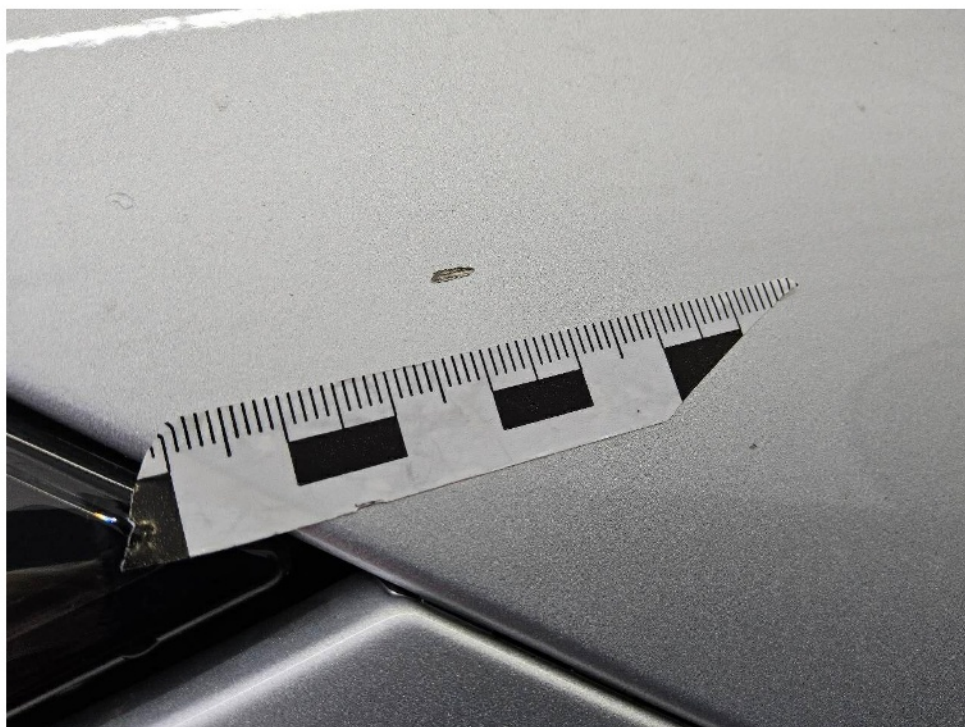
Bild 8 : Kotflügel vorn links bis auf das Grundmaterial verschrammt und eingedellt
