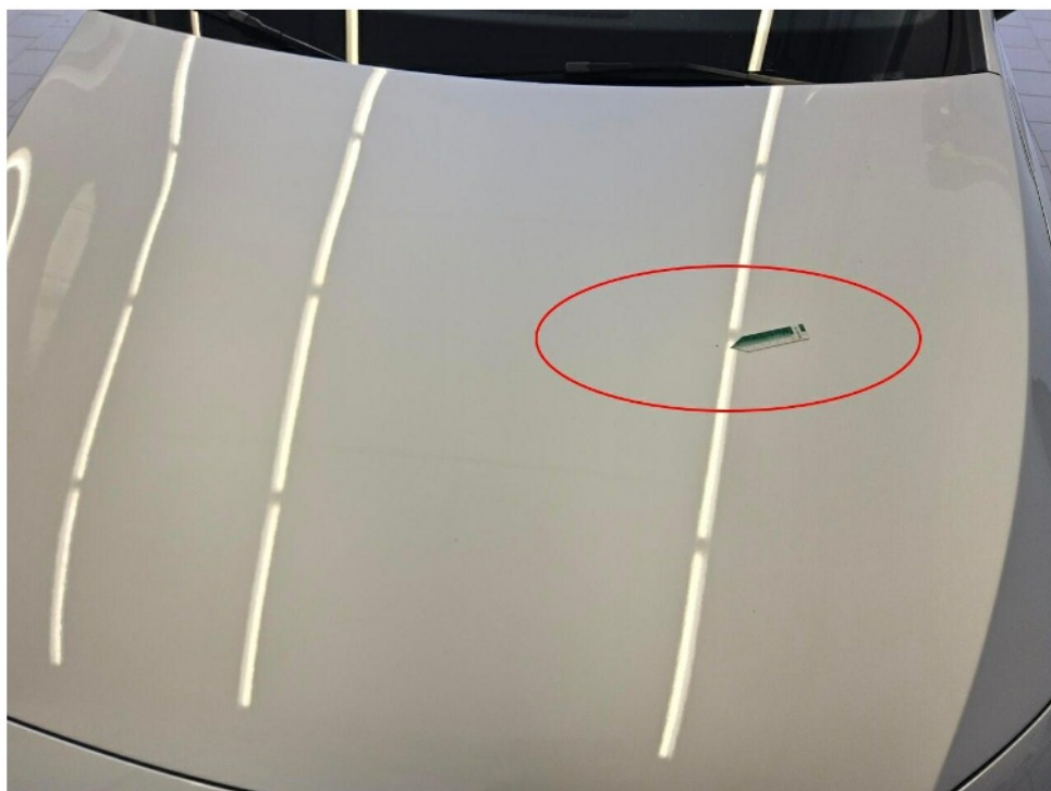
Bild 11 : Motorhaube Lackierung, Steinschlag, lackieren mit Lackaufbau
