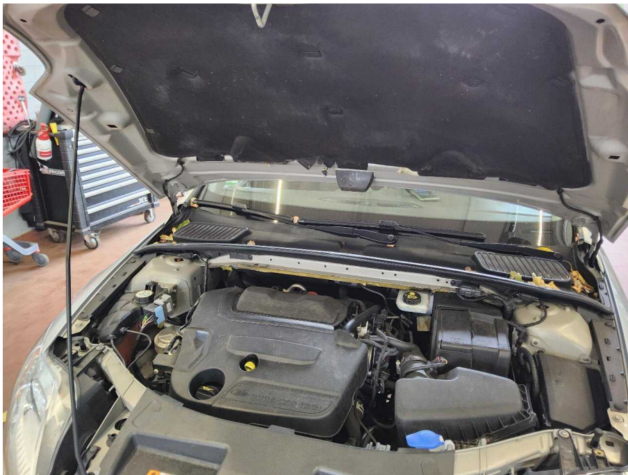
Bild 13: Motorraum
