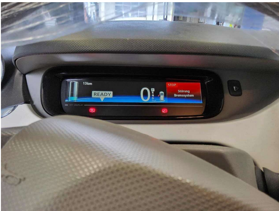
Bild 20 Systeme ABS ohne Funktion Fehlermeldung
