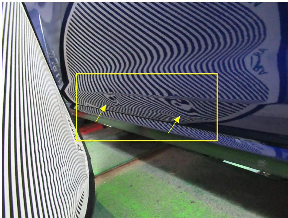
Bild 9 : Tür vorne unten links mehrfach eingedrückt
