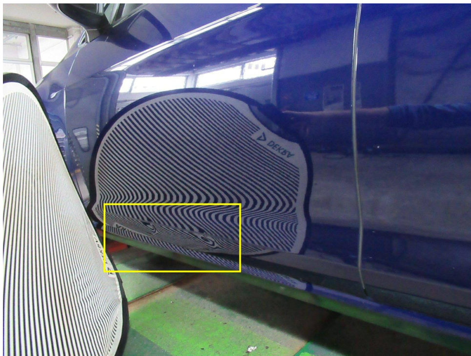
Bild 8 : Tür vorne unten links mehrfach eingedrückt
