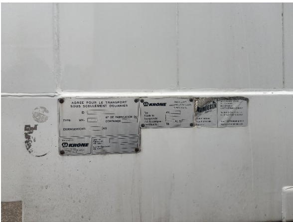
Bild 5: Typenschild
