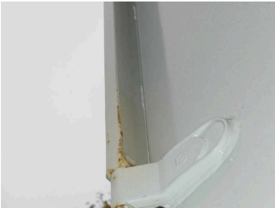
Bild 22 Fahrzeugheck Ecksäule hinten links deformiert
