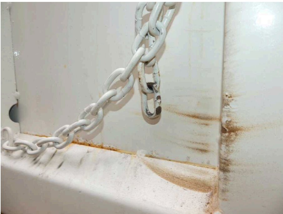
Bild 36 Fahrzeugheck Heckflügeltür links korrodiert
