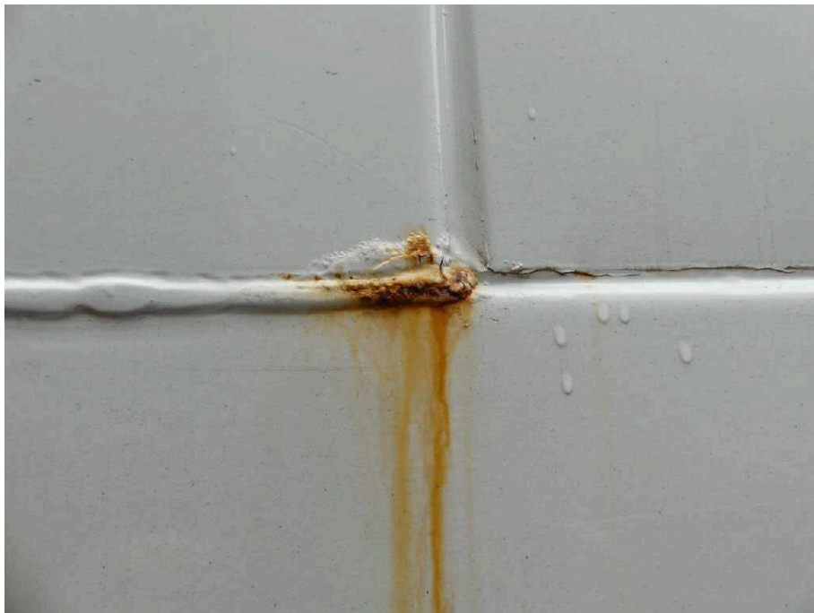
Bild 13 Fahrzeug Fahrzeug aussen links, verkratzt und korrodiert
