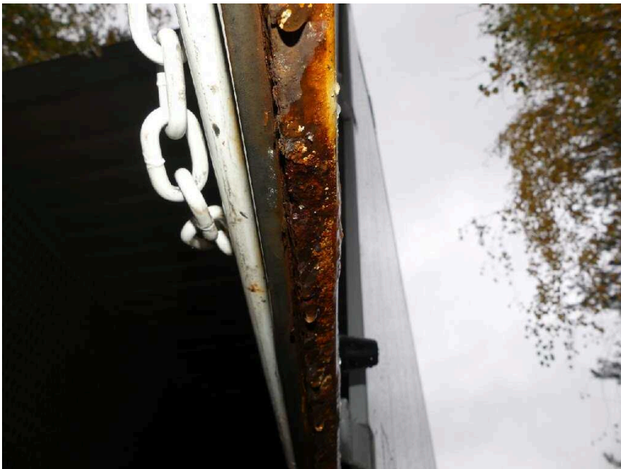
Bild 18 Fahrzeugheck Heckflügeltür rechts stark korrodiert
