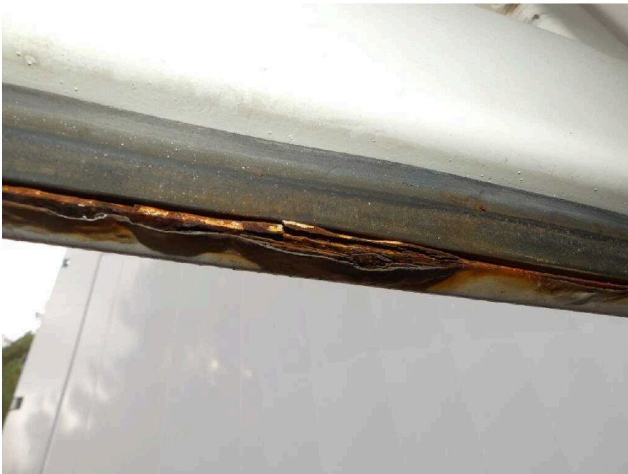
Bild 38 Fahrzeugheck Heckflügeltür links stark korrodiert
