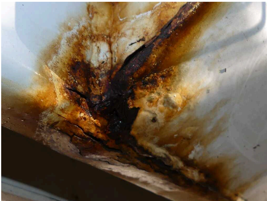
Bild 52 Fahrzeugheck Rahmen hinten rechts korrodiert
