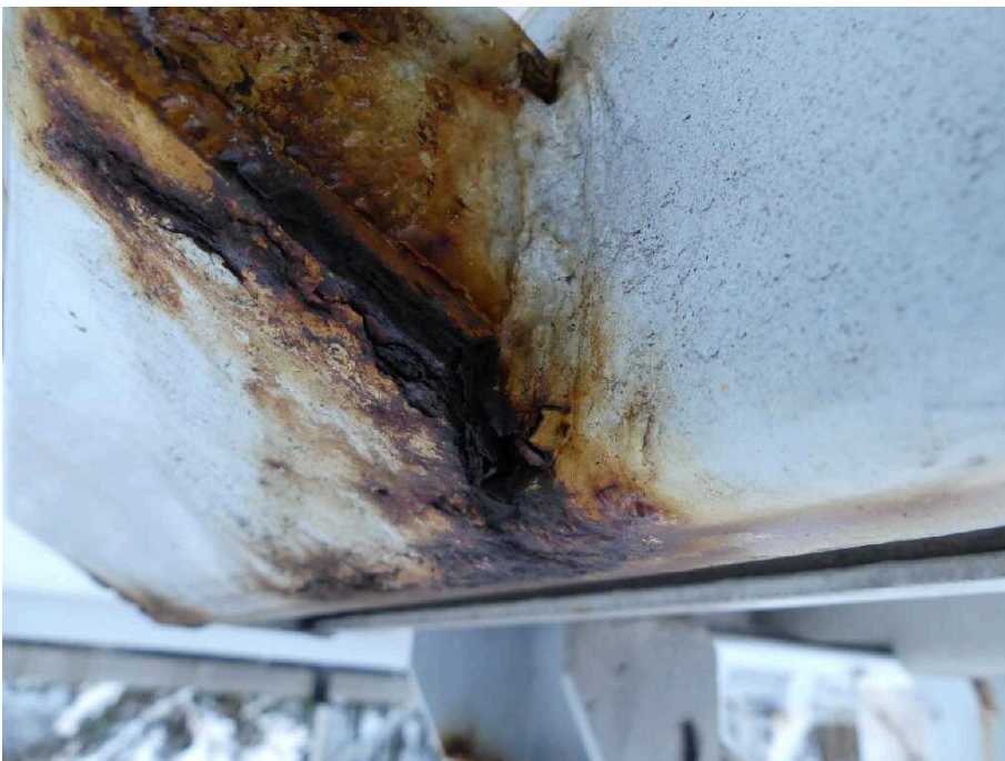
Bild 26 Fahrzeugheck Rahmen hinten hinten links stark korrodiert
