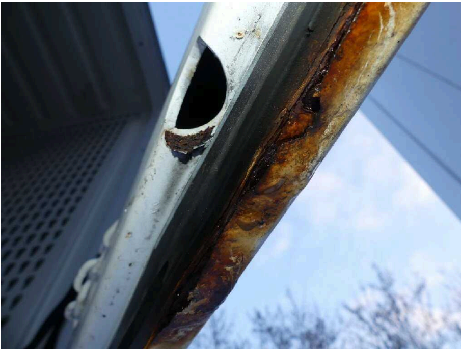
Bild 38 Fahrzeugheck Heckflügeltür rechts stark korrodiert
