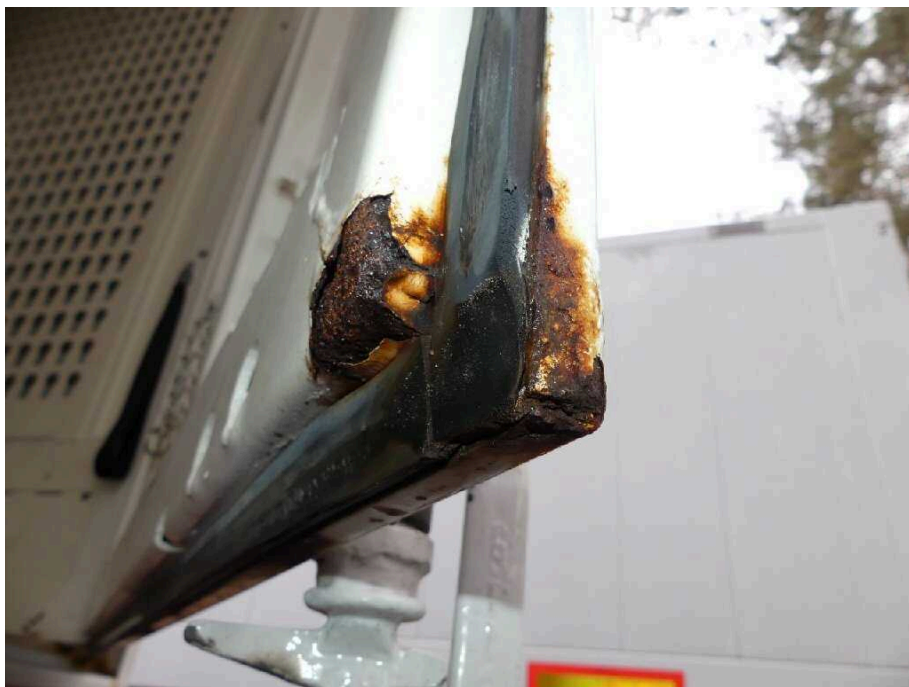
Bild 46 Fahrzeugheck Heckflügeltür links und rechts korrodiert
