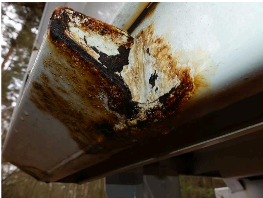
Bild 37 Fahrzeugheck Rahmen hinten links korrodiert
