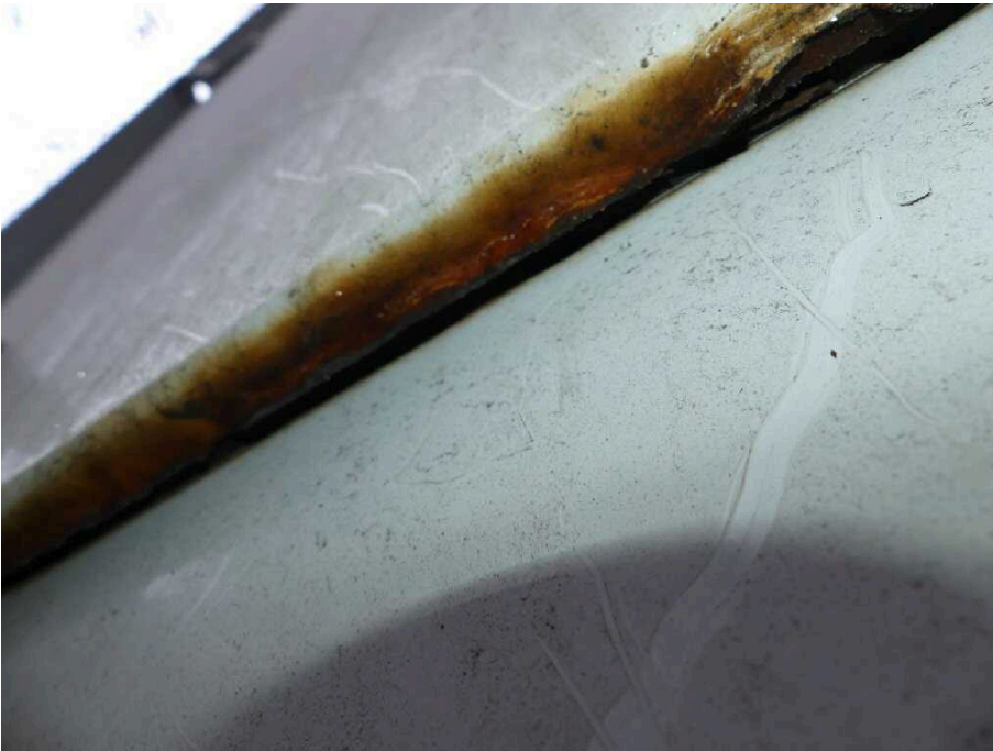
Bild 28 Fahrzeugheck Hecktür links stark korrodiert
