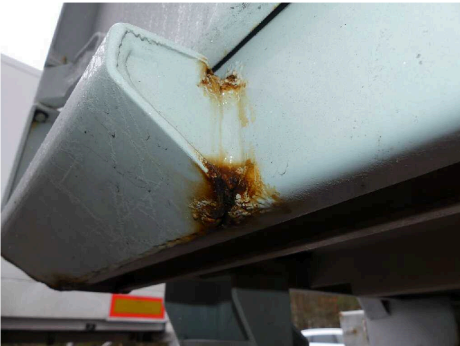
Bild 22 Fahrzeugheck Rahmen hinten links korrodiert
