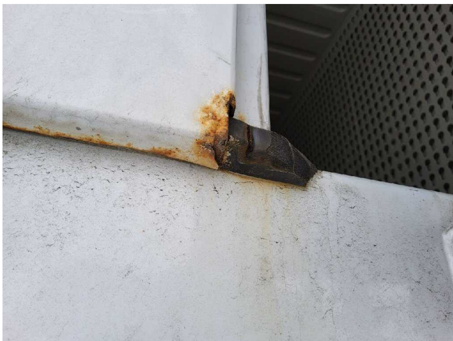
Bild 13 linke Seite Tür hinten links korrodiert
