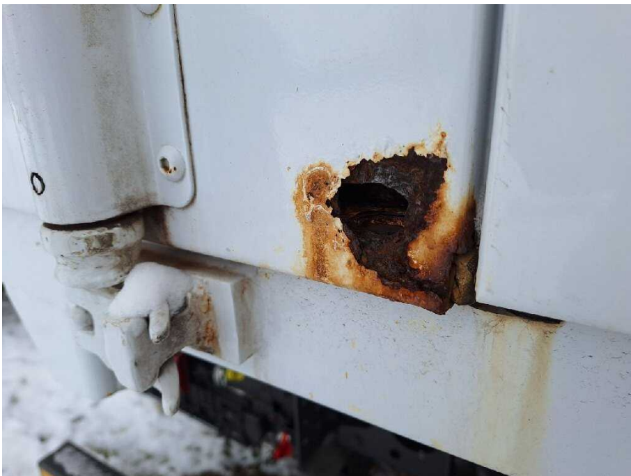
Bild 20 Fahrzeugheck Heckflügeltür links stark korrodiert
