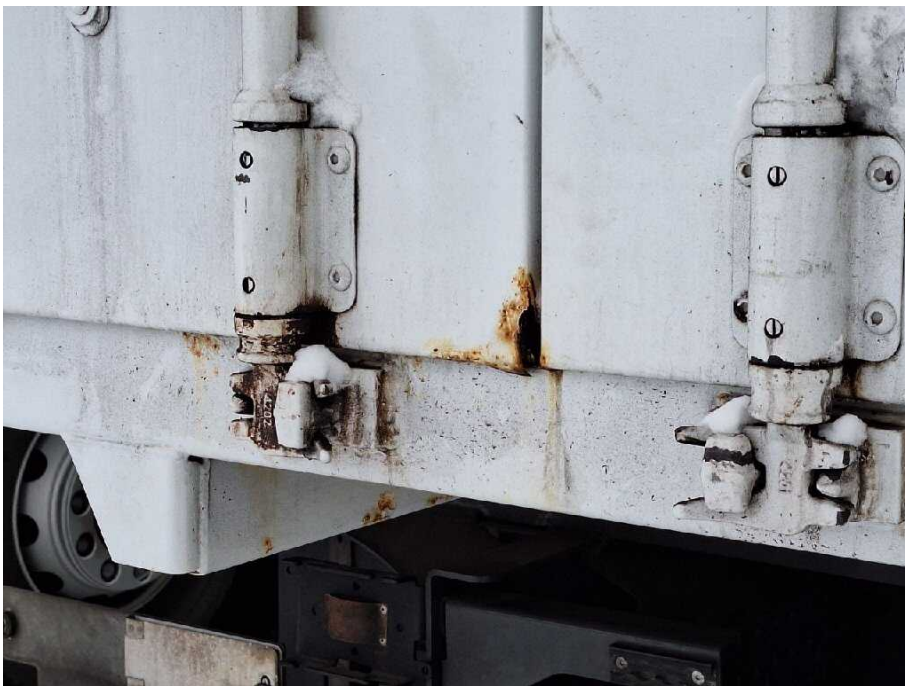
Bild 12 Fahrzeugheck Heckflügeltür links stark korrodiert
