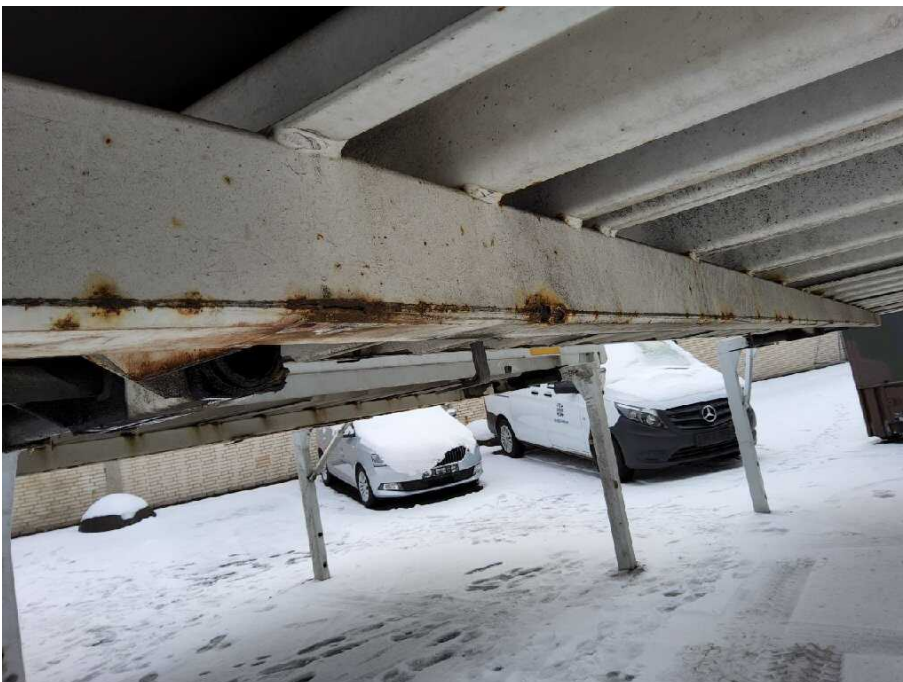
Bild 22 Aufbau Bodenrahmen hinten korrodiert
