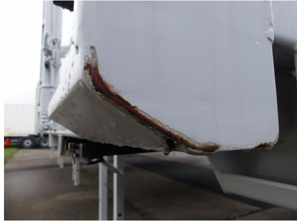
Bild 20: Eckbeplankung rechts Korrosion - instandsetzen und lackieren
