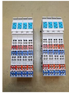
R-IB IL 24 DI 16-PAC Art.-Nr.: R911170752-101
