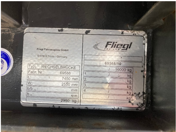
Bild 4: Typenschild
