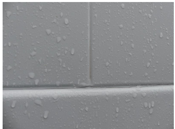
Bild 18: Abdichtung links und rechts beschädigt - erneuern
