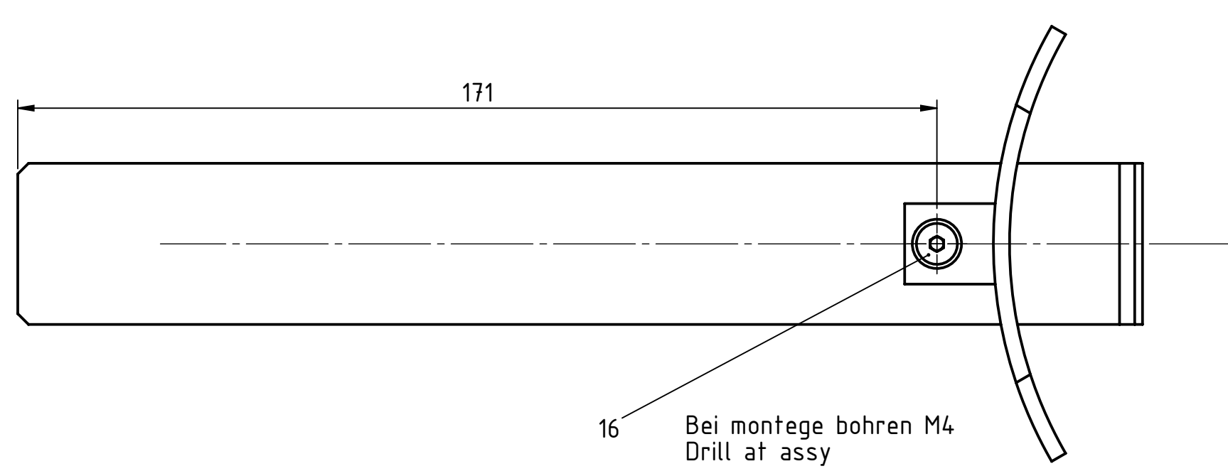
Schnitt / Section B-B
